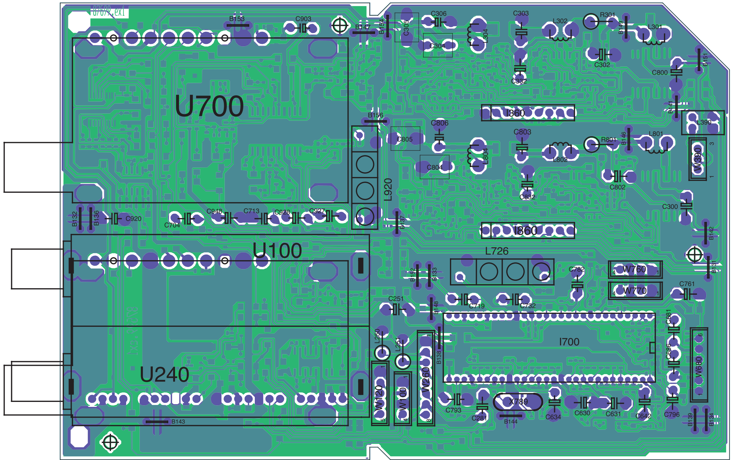
Leiterplatte SAT 6 87699E (Bestückungsseite)
